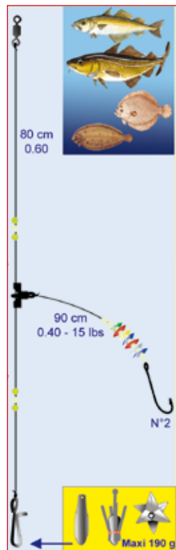
DL14 - Trainard coulissant
